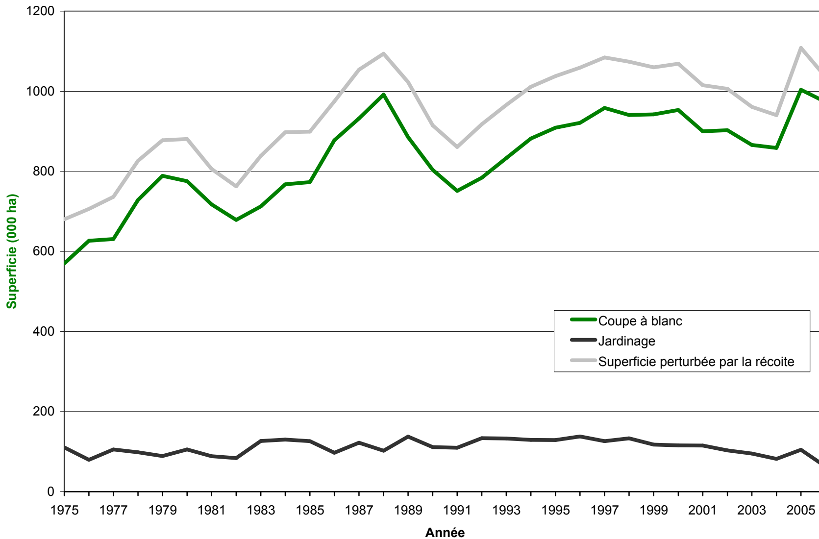
Figure 2.3c Superficies forestières perturbées par la récolte au Canada (1975–2006) (CCMF, 2008).
