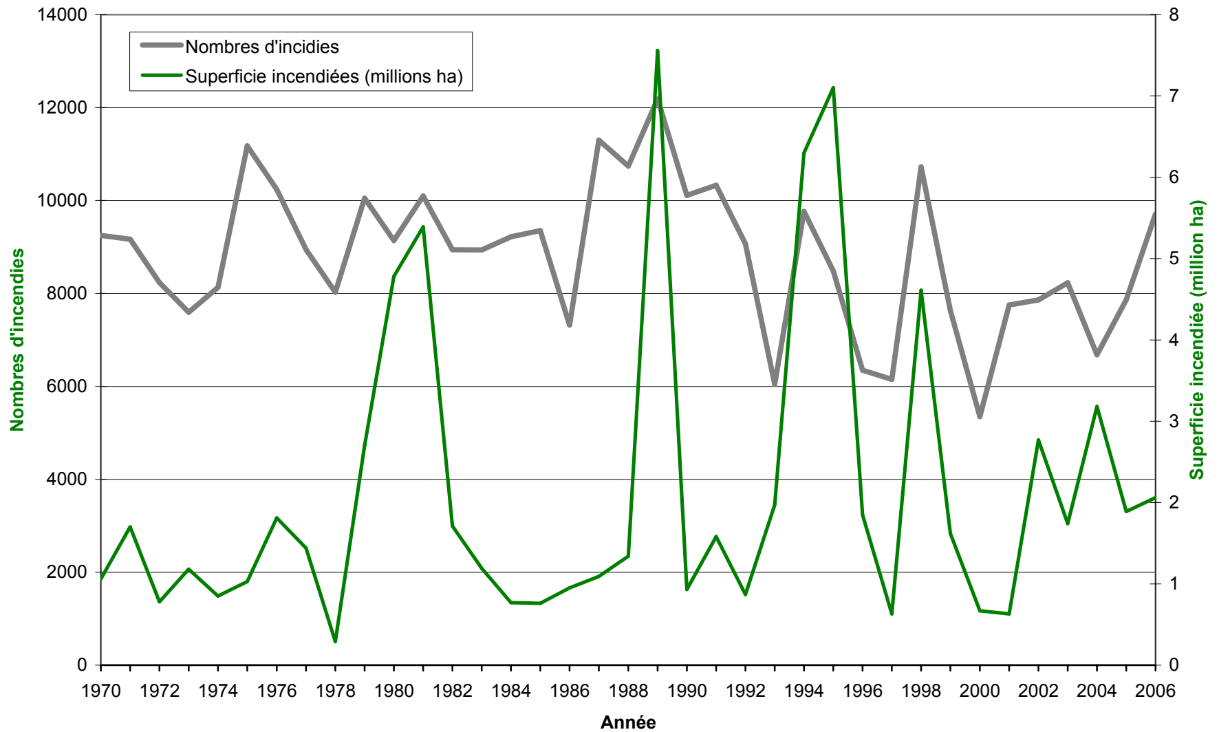
Figure 2.3a Nombres d'incidies de forêt et superficies incendiées au Canada (1970-2006) (CCFM, 2006; CFFI, 2008; Johnston, 2005)
